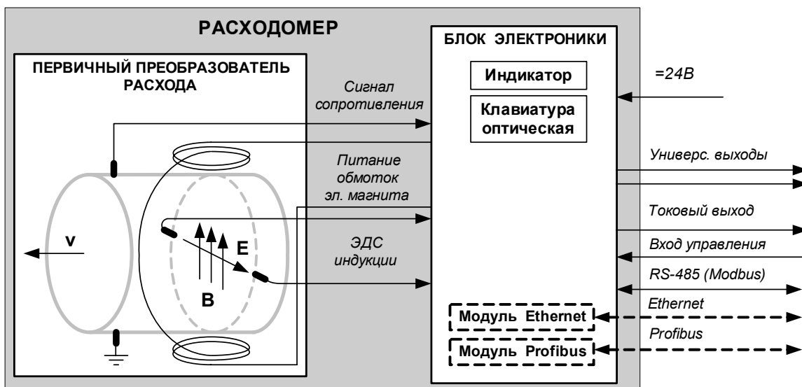
Рис.1. Структура расходомера.
