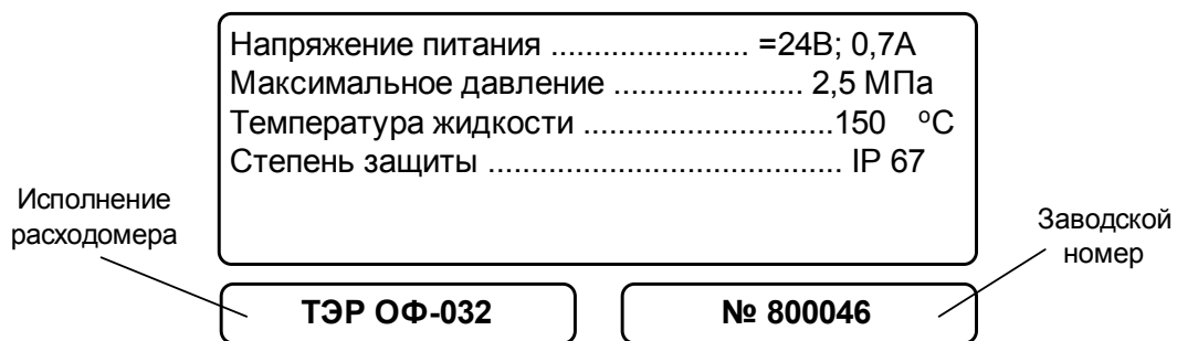
Рис.2. Вид шильда расходомера.
