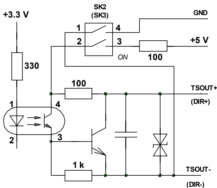
Рис.Б.1. Схема оконечного каскада универсальных выходов.
