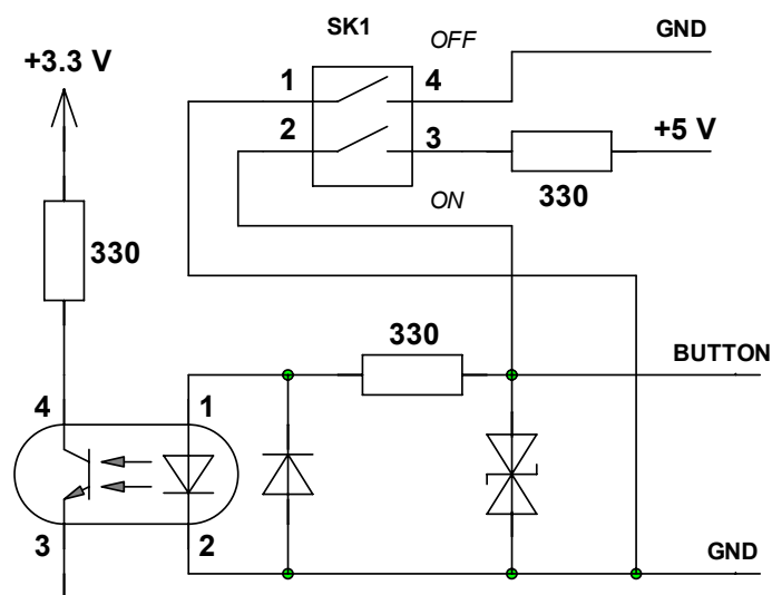
Рис.Б.3. Схема входного каскада расходомера.
