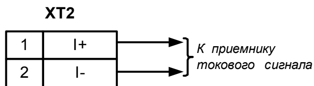
Рис.Б.2. Разъем ХТ2 токового выхода расходомера.
