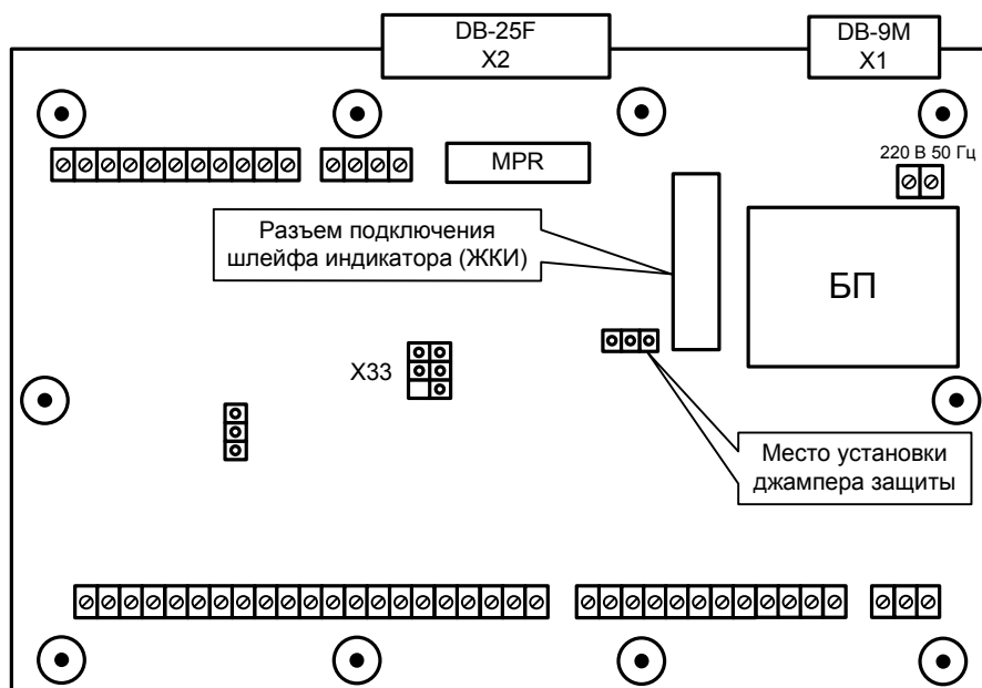
Рисунок 2. Расположение джампера в теплосчётчиках модификации «Т».
