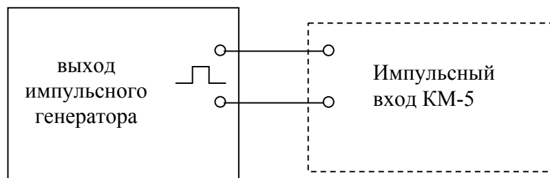
Рисунок П1.6. Схема проверки импульсных входов каналов объема (без преобразователей объема) при воспроизведении пакетов импульсов с помощью импульсного генератора
