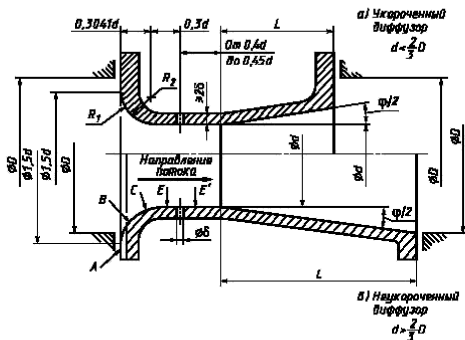
Рисунок 9 — Сопло Вентури
