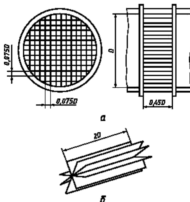
Рисунок 2 — Струевыпрямители
