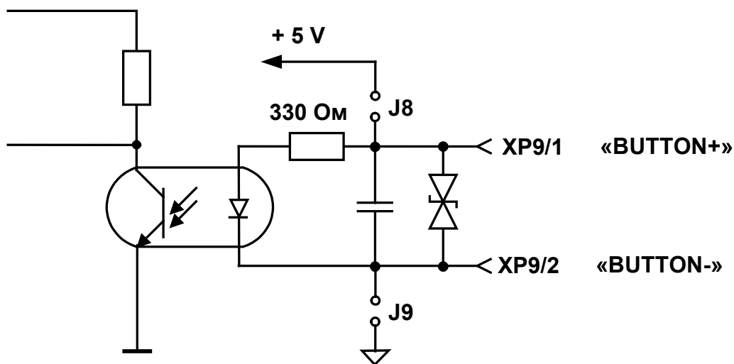
Рис. Б.4. Схема входного каскада БВИ.
