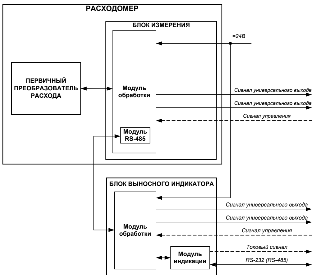
Рис. 4. Функциональная схема расходомера исполнения ПРОФИ-3xx.
