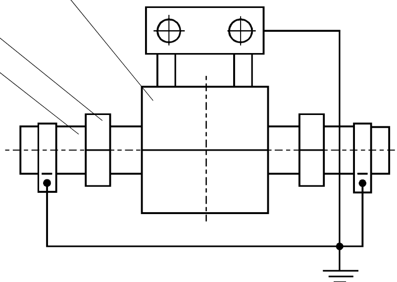
Рисунок 18 - Схема заземления первичных преобразователей
