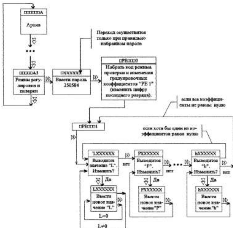
Схема проверки и изменения градуировочных коэффициентов
