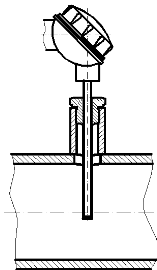
Рисунок Г.3 — Вертикальная установка термопреобразователя
