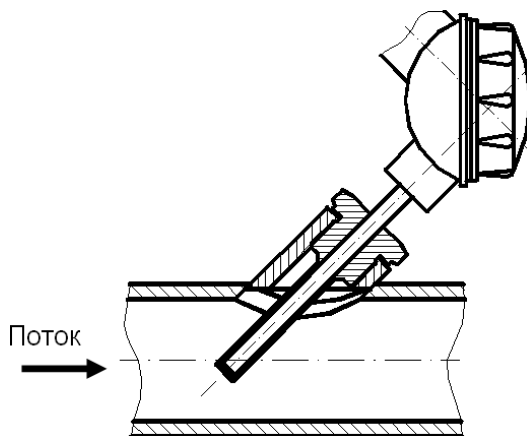
Рисунок Г.4 — Наклонная установка термопреобразователя
