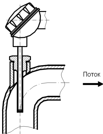
Рисунок Г.5 — Установка термopеобразователя в колено
